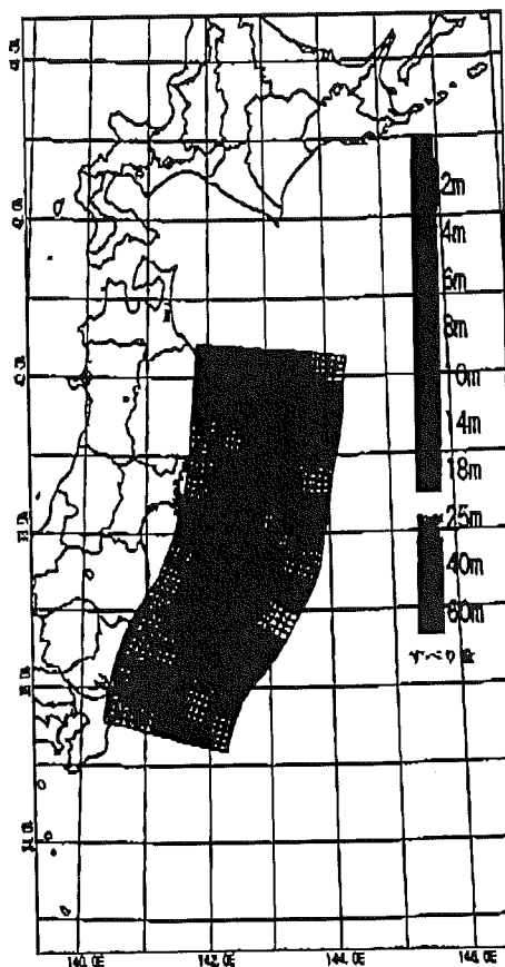
今回の津波の波源 (東京電力作成 1 )
